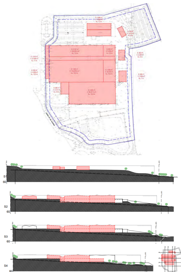
Plànol i seccions de la ubicació actual de l'edificació. Font: MPPGO art.159
