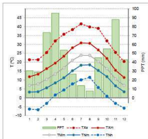
Figura 23. Normals climàtiques a l'estació meteorològica de Falset (2007-2016).
