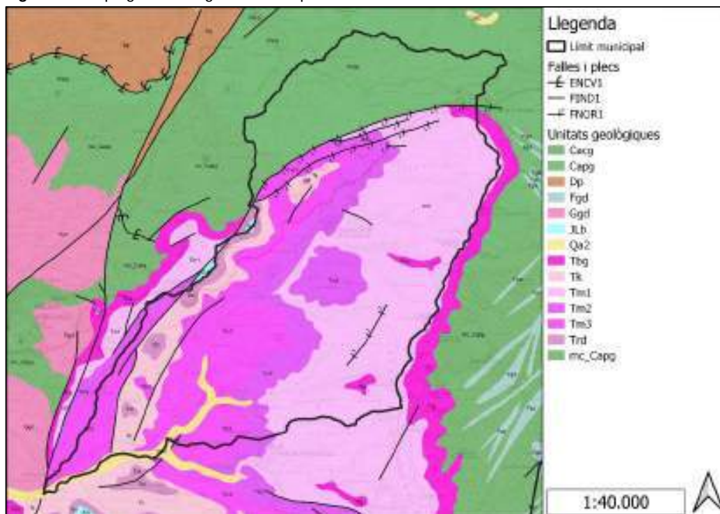
Figura 20. Mapa geomorfològic del municipi de Pradell de la Teixeta.
