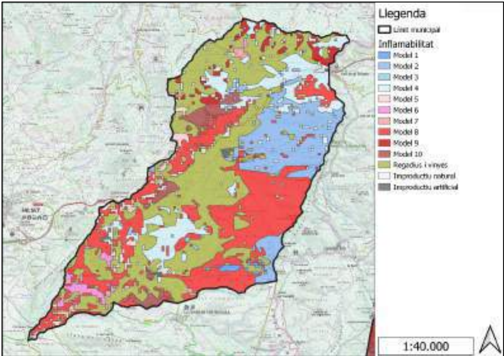
Figura 11. Models d'inflamabilitat en el municipi de Pradell de la Teixeta.
