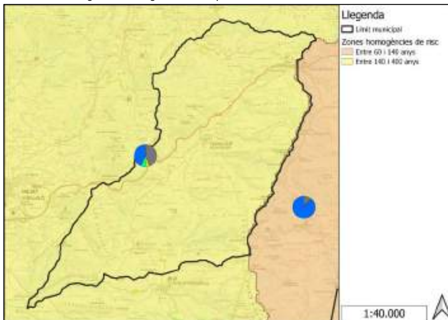
Figura 19. Zones homogènies de règim al municipi de Pradell de la Teixeta.
