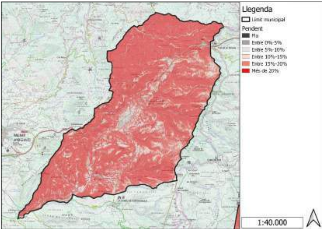
Figura 4. Distribució dels pendents al terme municipal de Pradell de la Teixeta.
