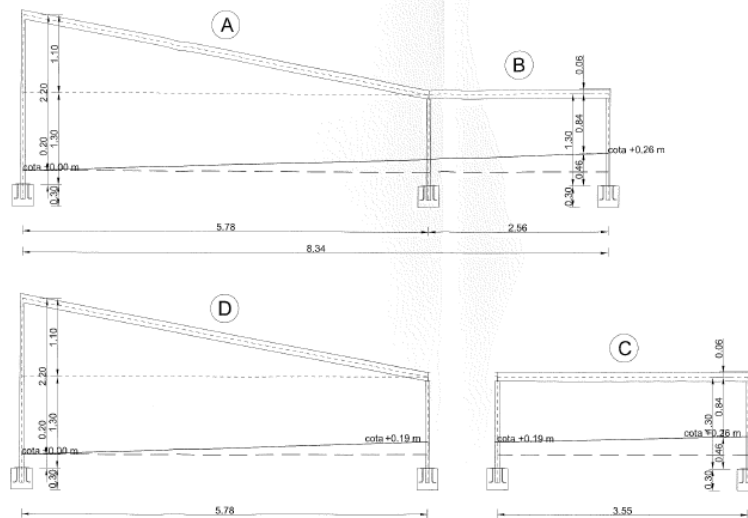
SECCIONS PERFILS GRUP 1 e:1/25
