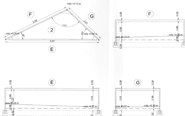
PLANTA I SECCIONS PERFILS GRUP 2 e:1/25
